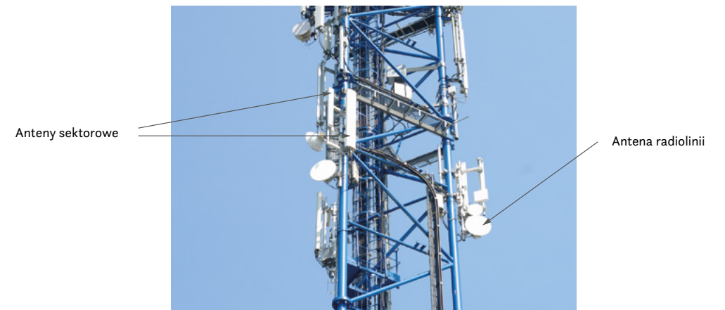
Rys. 4. Rodzaje anten w stacji bazowej telefonii komórkowej. Źródło: własne IŁ-PIB
