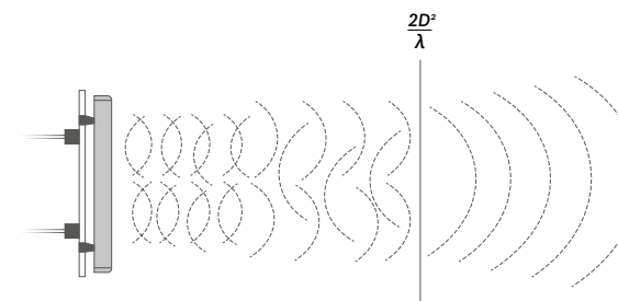
Rys. 1. Zobrazowanie strefy bliskiej i dalekiej. Autor: Paweł Woźniak
